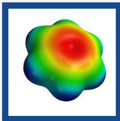
Benzene
